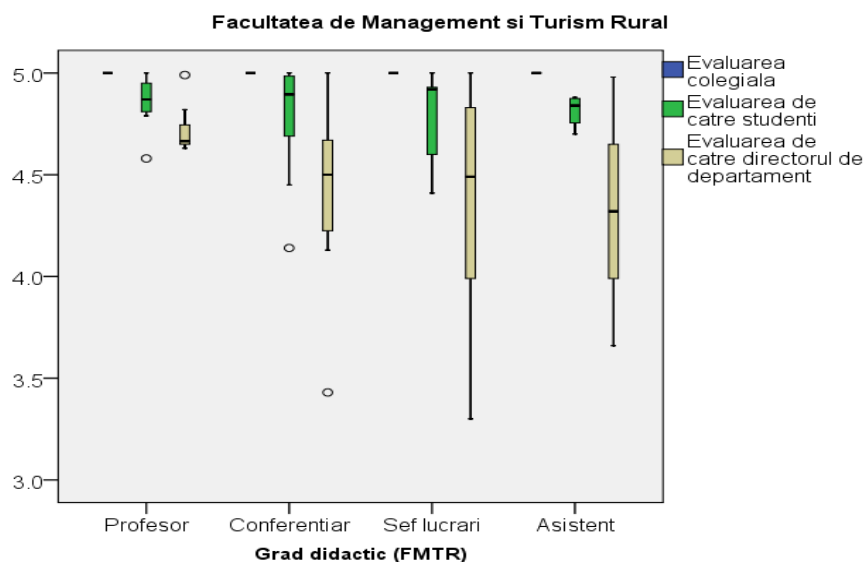
Figura 3. ,Diagrama boxplot aferentă punctajelor obținute de cadrele didactice la evaluarea colegială, la evaluarea de către studenți, respectiv la evaluarea de către directorul de departament
