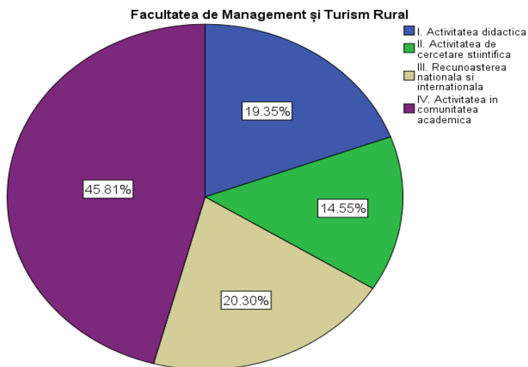
Figura 1. Ponderea criteriilor din fișa de autoevaluare
